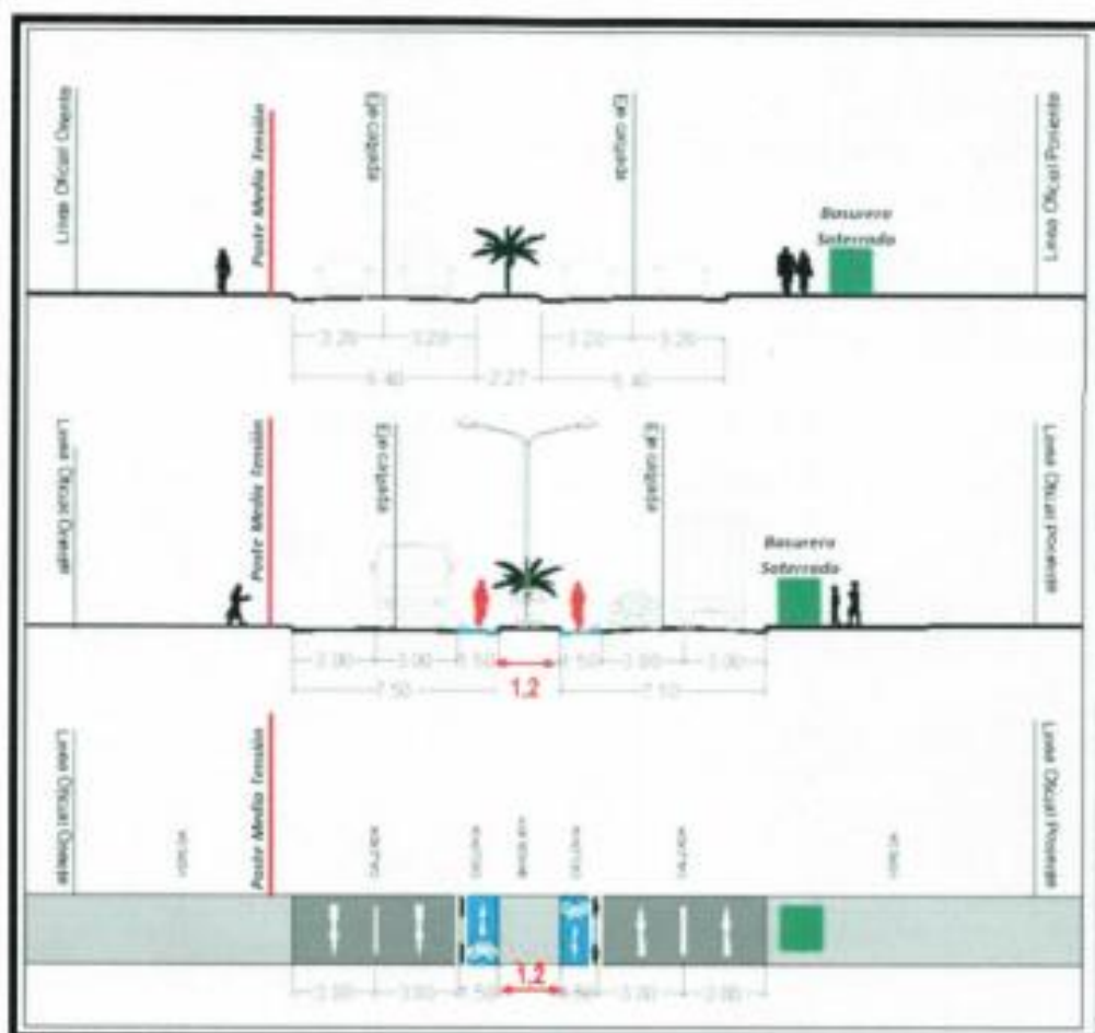
Imagen 3: Perfil modificado, bandejón pasa de 2,27 a 1,2m.
