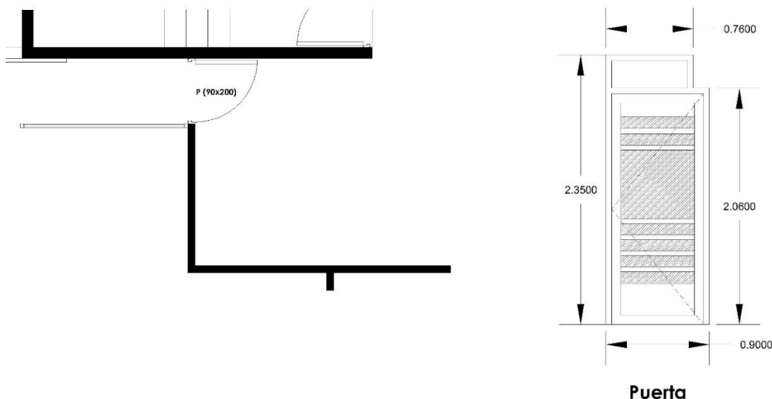
Fig. 03. Planta y elevación puerta.
